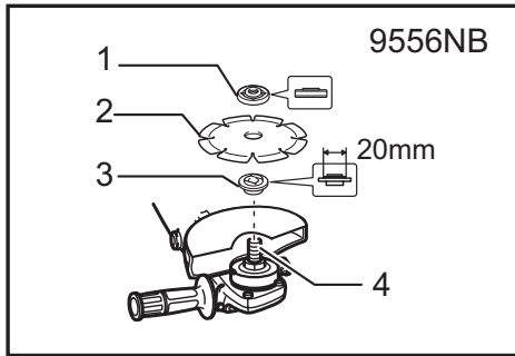
► 1. Contratuercia 2. Disco de diamante 3. Brida interior 4. Eje
