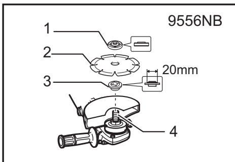
► 1. Lock nut 2. Diamond wheel 3. Inner flange 4. Spindle
